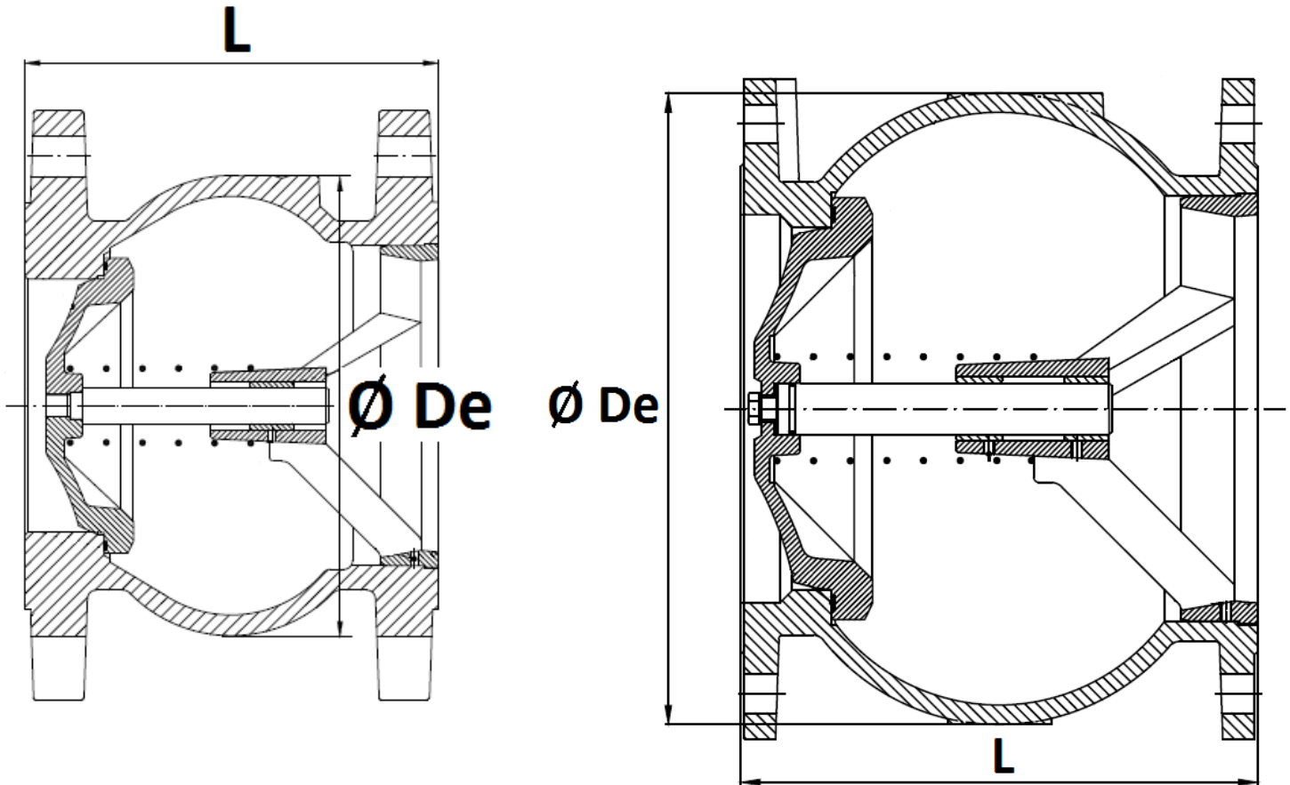
DN50 – 100
